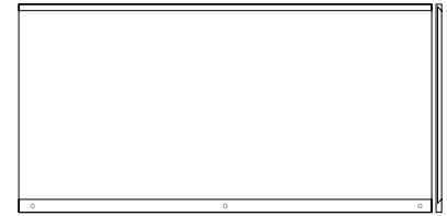
par 363 V w 630 x h 318 x d 9,5mm w 24,8 x h 12,52 x d 0,37"
